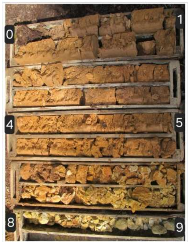
Jádrový vrt JV1, 0 - 9 m
